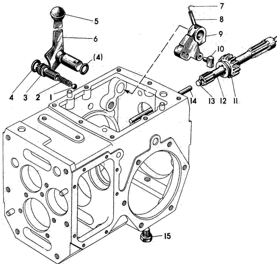
Рисунок 11 – Управление и привод ВОВ
