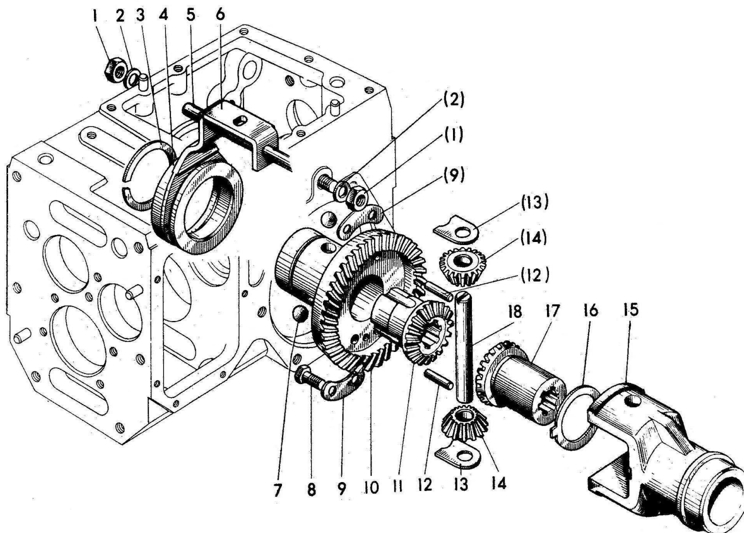
Рисунок 6 – Дифференциал
