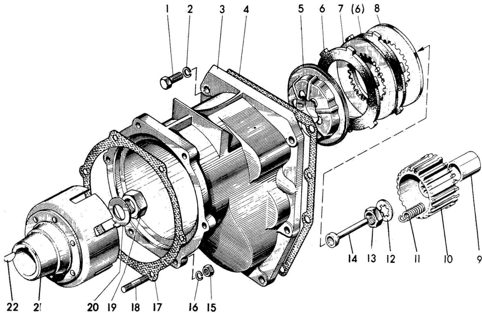
Рисунок 2 – Сцепление
