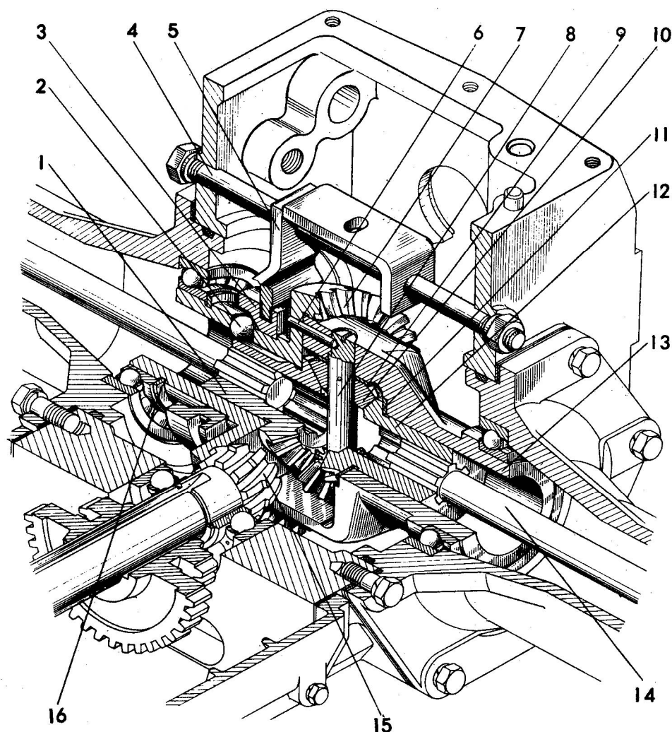
Рисунок 11 – Ведущий мост
