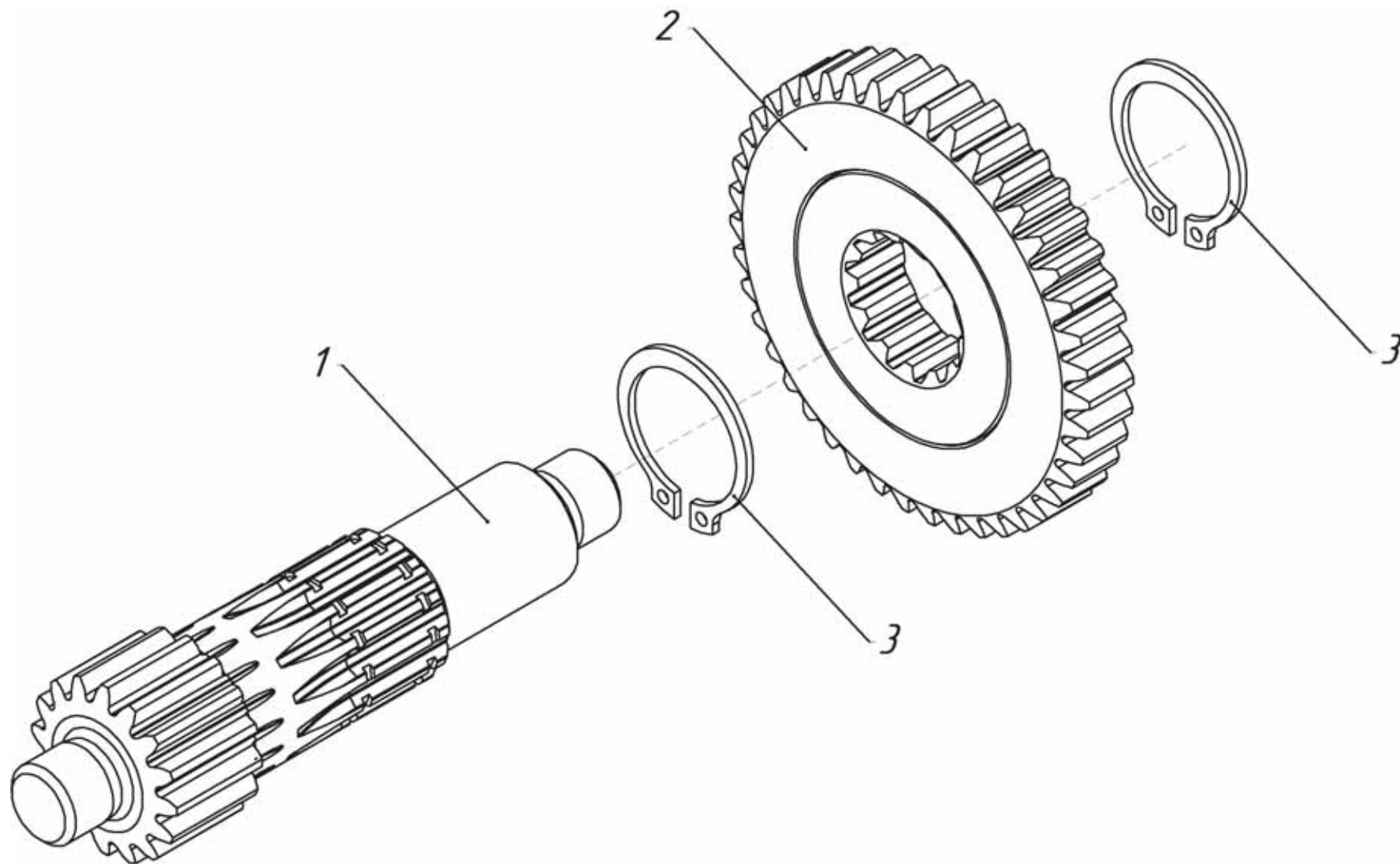
Рис.13 (005.65.0450 Вал промежуточный)
